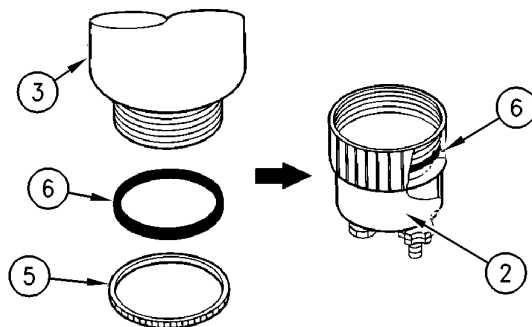
Рисунок 2 (2) Стакан водоотделителя (3) Фильтр (5) Крышка (6) Уплотнение
