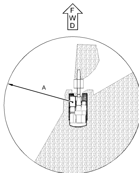
Рисунок 1 Вид машины сверху, обзор с уровня земли без использования дополнительных средств улучшения обзора (A) 12 m (39 ft)
