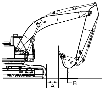
Рисунок 3 g02155813 (A) 1 m (3.0 ft) от передней части машины до ковша (B) 0.5 m (1.6 ft) от уровня земли
