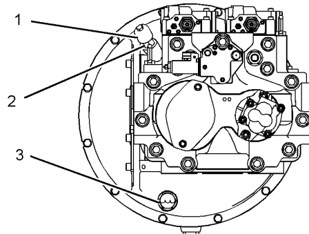
Рисунок 1 (1) Салун (2) Переходник (3) Смотровой указатель
