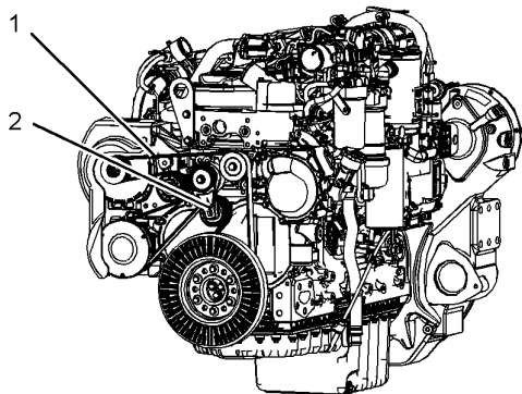
Рисунок 1 Модель 120М серии 2
