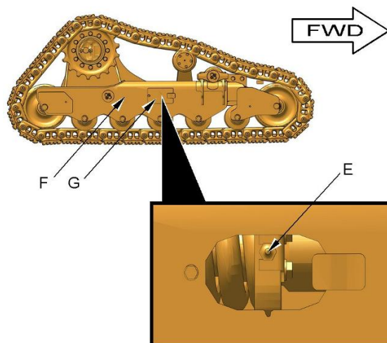
Рисунок 2 (E) Смазочный клапан - группа натяжителя (F) Правая ходовая часть в сборе (G) Пластина крышки смазочного клапана группы натяжителя
