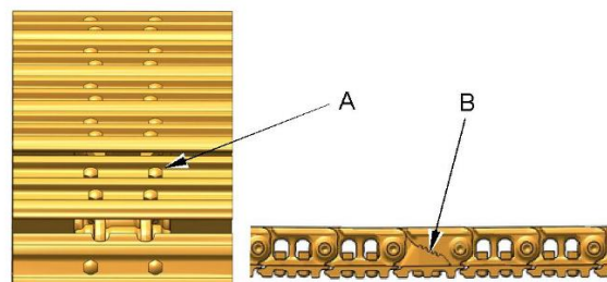
Рисунок 3 (A) Болты грунтозацепа гусеничной ленты (B) Болты главных звеньев
