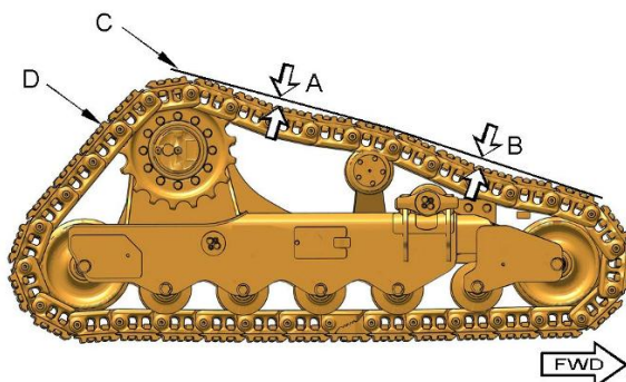
Рисунок 1 g06324053 (A) Первая точка измерения (B) Вторая точка измерения (C) Контрольный шнур (D) Профиль гусеничной ленты
