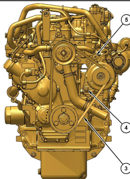
Рисунок 2 C2.2 (3) Клиновой ремень (4) Болт крепления генератора (5) Регулировочный болт g06387503
