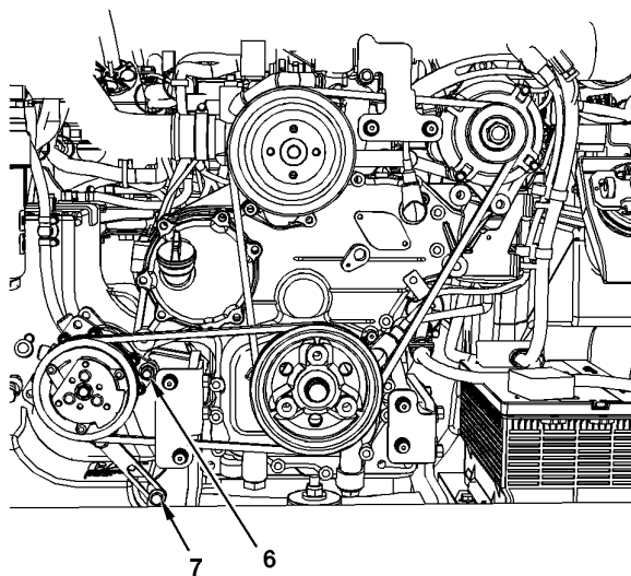
Рисунок 8 СЗ.8 (6) Монтажный болт (7) Регулировочный болт
