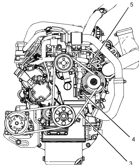
Рисунок 2 C2.2 g03820567 (3) Клиновой ремень (4) Болт крепления генератора (5) Регулировочный болт
