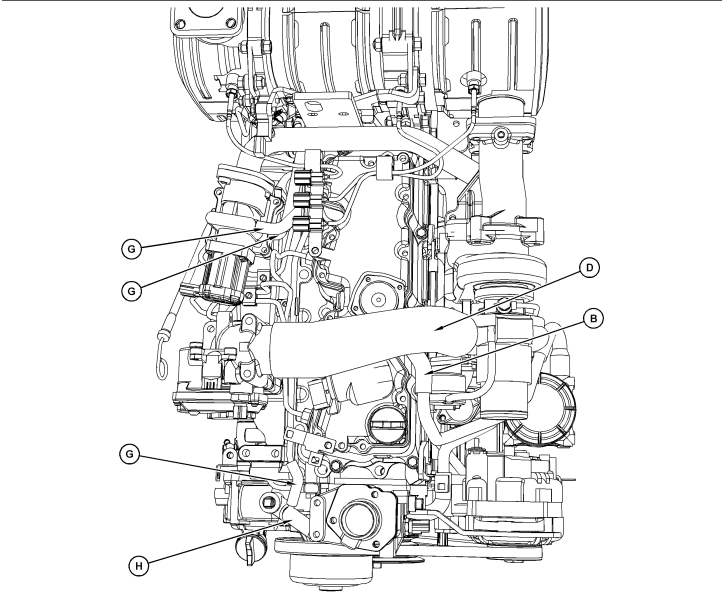
Рисунок 2 Вид сверху C3.8 g03818658
