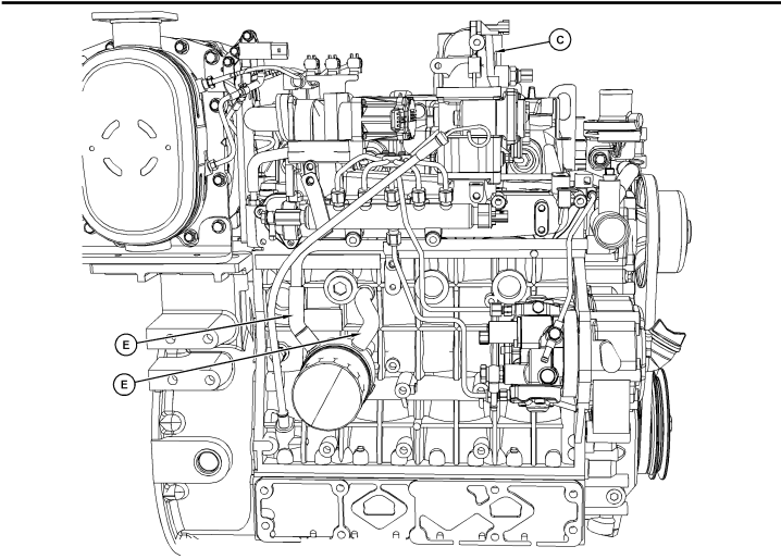
Рисунок 1 Левая сторона C3.8 g03818641
