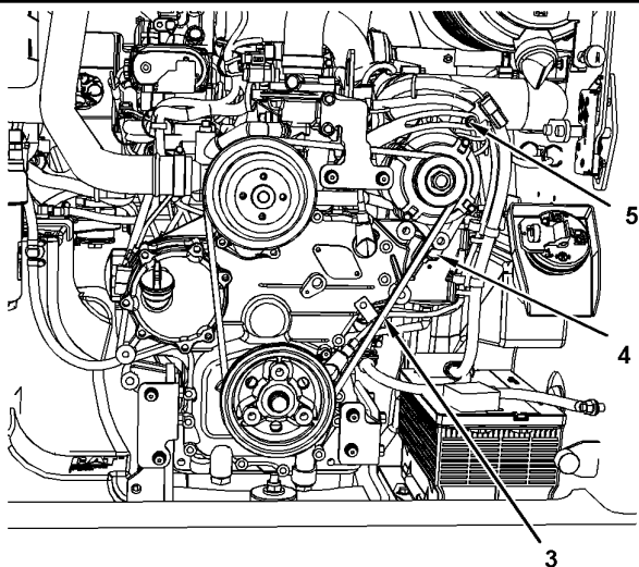
Рисунок 4 C3.8 (3) Клиновой ремень (4) Болт крепления генератора (5) Регулировочный болт
