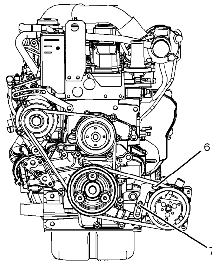
Рисунок 7 C3.3B (6) Монтажный болт (7) Регулировочный болт
