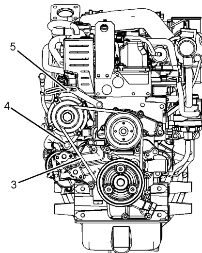
Рисунок 3 C3.3B g03384275 (3) Клиновой ремень (4) Болт крепления генератора (5) Регулировочный болт
