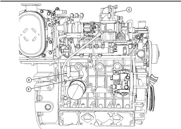
Рисунок 1 Левая сторона C3.8
