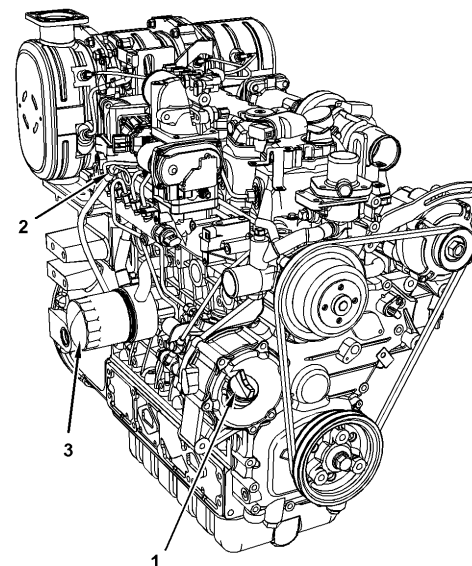
Рисунок 4 Двигатель C3.8 (1) Крышка маслоналивной горловины (2) Масляный щуп (3) Масляный фильтр
