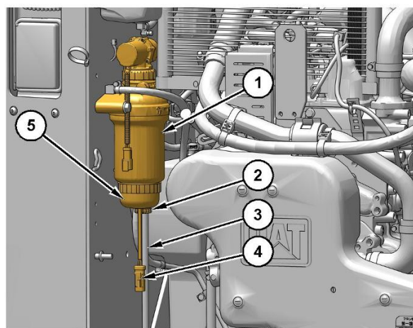
Рисунок 1 (1) Fuel Filter (2) Сливной клапан (3) Сливной шланг (4) Заглушка датчика присутствия воды в топливе (5) Водяной стакан
