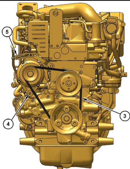
Рисунок 3 C3.3B (3) Клиновой ремень (4) Болт крепления генератора (5) Регулировочный болт
