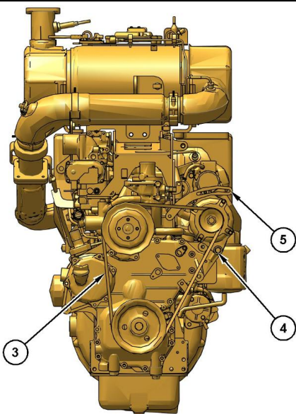
Рисунок 4 C3.8 (3) Клиновой ремень (4) Болт крепления генератора (5) Регулировочный болт
