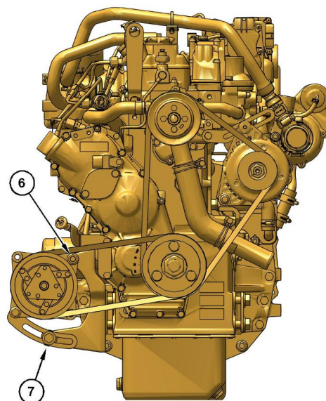
Рисунок 6 C2.2 (6) Монтажный болт (7) Регулировочный болт
