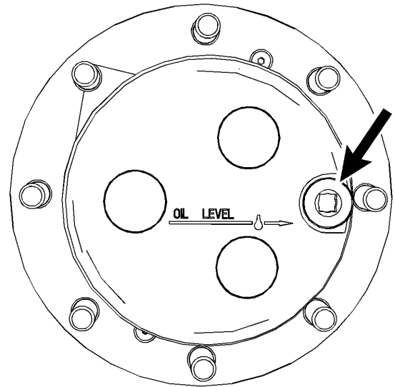
Рисунок 3 g01357831 Колесо в положении для проверки
