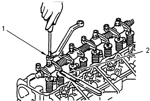
Рисунок 1 Настройка клапанного зазора (1) Регулировочный винт (2) Измерительный щуп
