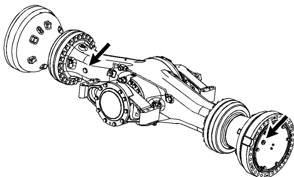
Рисунок 2 Задний мост
