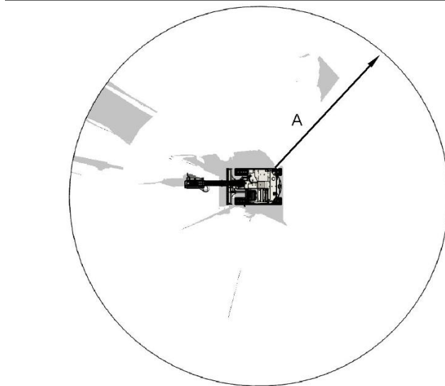
Рисунок 8 Машина, вид сверху Обзорность на уровне земли при наличии зеркала на противовесе, зеркала в кабине и камеры заднего вида. (A) 12 m (39 ft)
