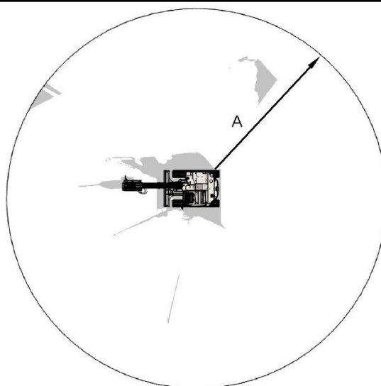
Рисунок 5 Машина, вид сверху Обзорность на уровне земли при наличии зеркала на противовесе, зеркала в кабине и камеры заднего вида. (A) 12 m (39 ft)
