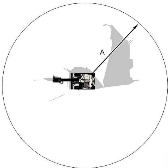
Рисунок 6 Машина, вид сверху Обзорность на уровне земли при наличии зеркала на противовесе и зеркала в кабине. (A) 12 m (39 ft)
