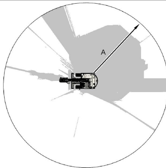
Рисунок 4 Машина, вид сверху Обзорность на уровне земли при отсутствии средств улучшения обзорности. (A) 12 m (39 ft)
