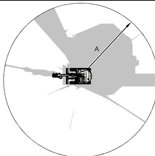
Рисунок 13 Машина, вид сверху Обзорность на уровне земли при отсутствии средств улучшения обзорности. (A) 12 m (39 ft) g06373532
