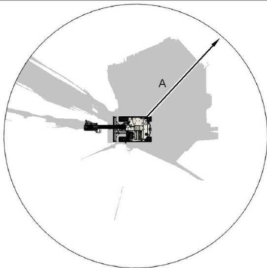
Рисунок 10 Машина, вид сверху Обзорность на уровне земли при отсутствии средств улучшения обзорности. (A) 12 m (39 ft) g06371899
