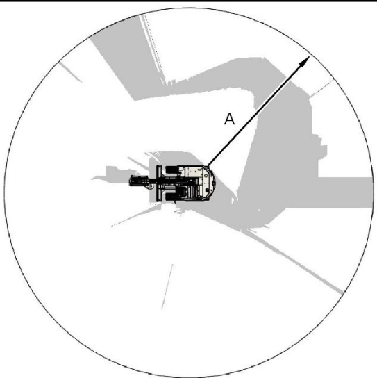
Рисунок 3 Машина, вид сверху Обзорность на уровне земли при наличии зеркала на противовесе и зеркала в кабине. (A) 12 m (39 ft)
