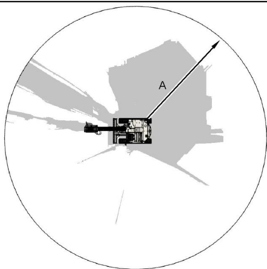
Рисунок 7 Машина, вид сверху Обзорность на уровне земли при отсутствии средств улучшения обзорности. (A) 12 m (39 ft)
