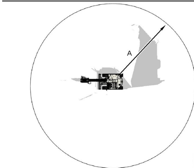
Рисунок 9 Машина, вид сверху Обзорность на уровне земли при наличии зеркала на противовесе и зеркала в кабине. (A) 12 m (39 ft)
