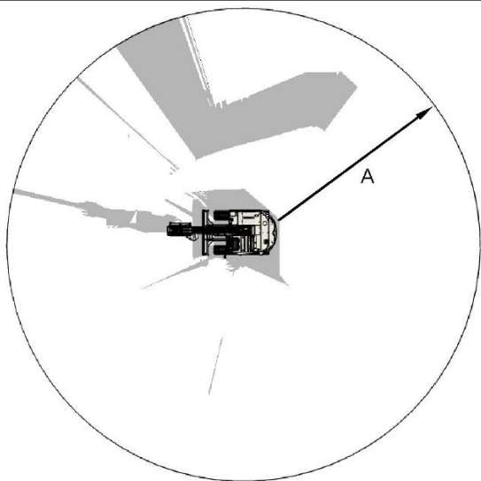
Рисунок 2 Машина, вид сверху Обзорность на уровне земли при наличии зеркала на противовесе, зеркала в кабине и камеры заднего вида. (A) 12 m (39 ft)
