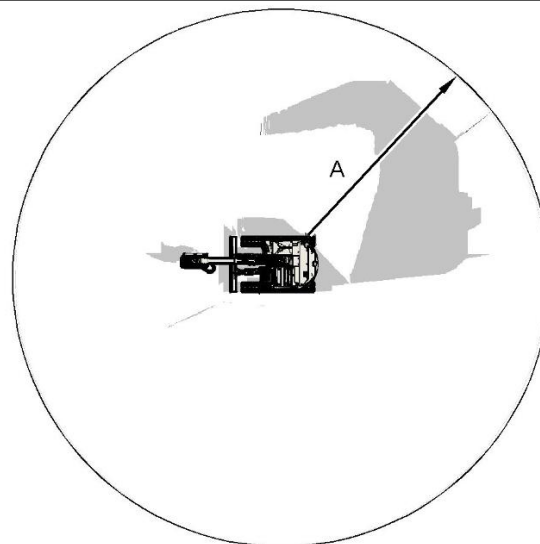
Рисунок 12 Машина, вид сверху Обзорность на уровне земли при наличии зеркала на противовесе и зеркала в кабине. (A) 12 m (39 ft) g06373531
