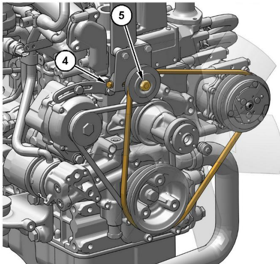
Рисунок 4 (4) Регулировочный болт (5) Монтажный болт
